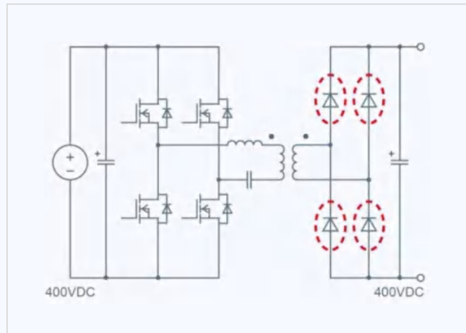
二次侧整流电路
